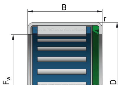
HK...RS
