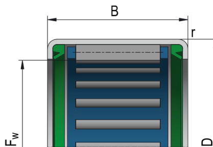
HK...2RS
