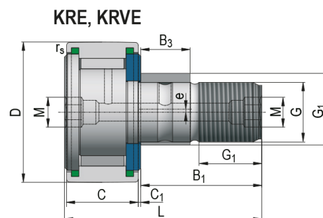
KRE..PP, KRVE..PP
